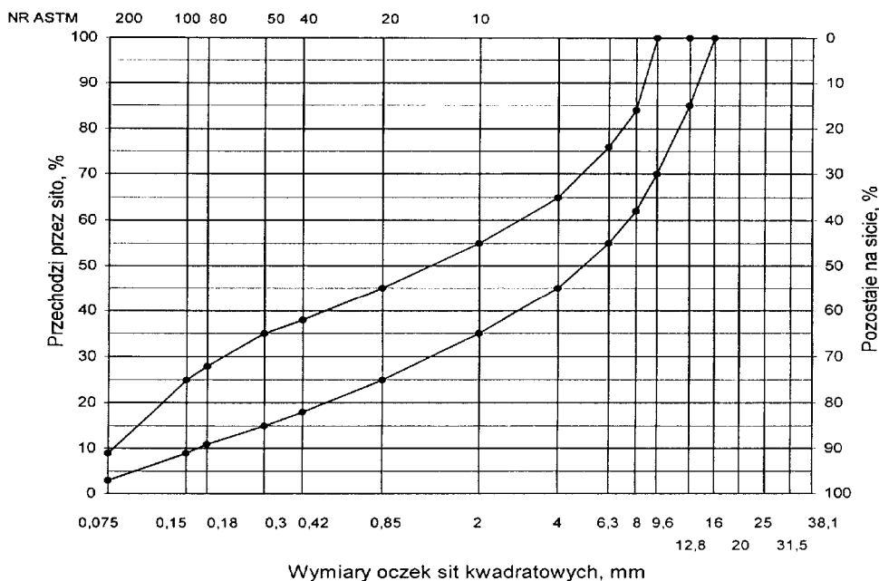
Rys. 2. Krzywe graniczne uziarnienia mieszanki mineralnej BA od 0 do 12,8 mm do warstwy wiążącej
