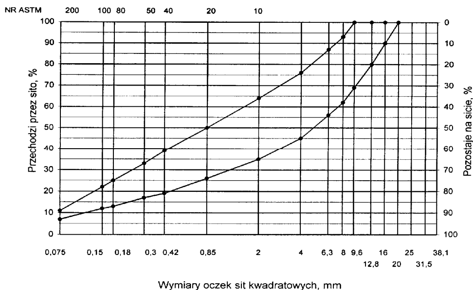
Rys. 1. Krzywe graniczne uziarnienia mieszanki mineralnej BA od 0 do 12,8 mm do warstwy ścieralnej nawierzchni drogi
