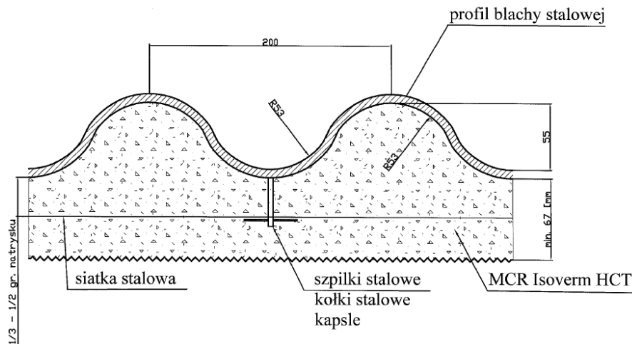
Rys.3 Zabezpieczenie powierzchni tunelu z blachy falistej
