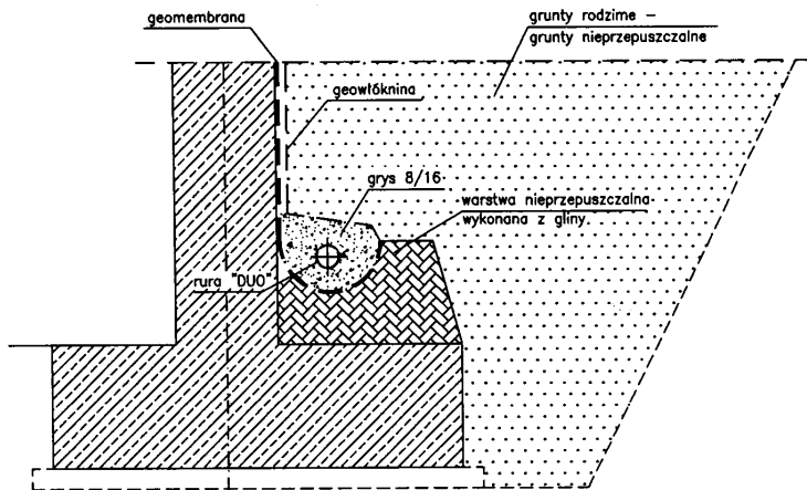
Rys. 1. Warstwa filtracyjna za ścianą z tworzywa sztucznego
