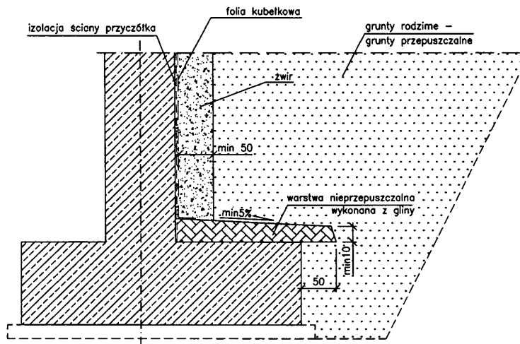
Rys. 2. Warstwa filtracyjna za ścianą z folii i warstwy żwiru
