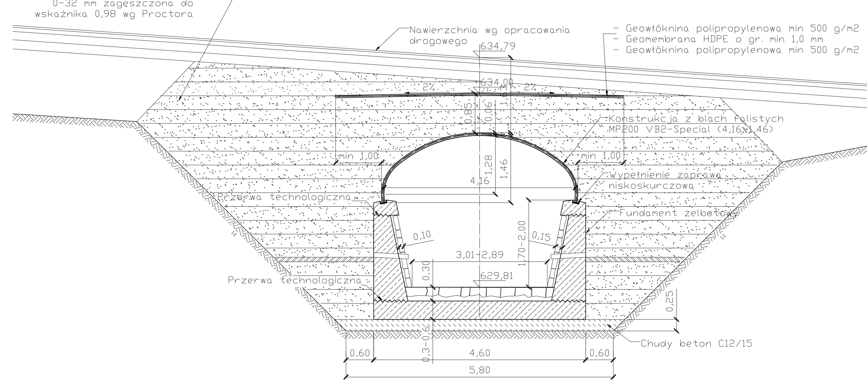
Przekrój poprzeczny A-A
