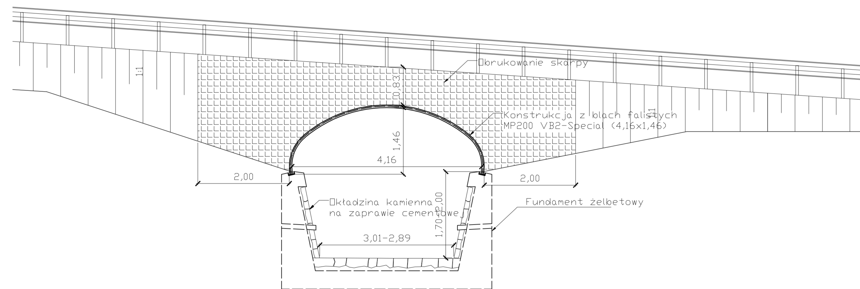
Widok z boku (wlot) C-C
