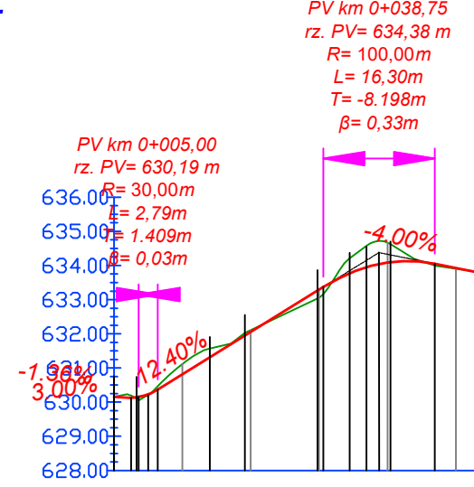
PRZEKRÓJ PODŁUŻNY UL. ZJAZD WYSPIAŃSKIEGO km 0+382 km 0+000,00 do km 0+055,54 SKALA 1:1000/200
