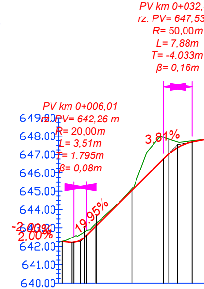
PRZEKRÓJ PODŁUŻNY UL. ZJAZD WYSPIAŃSKIEGO km 0+072 km 0+000,00 do km 0+040,88 SKALA 1:1000/200
