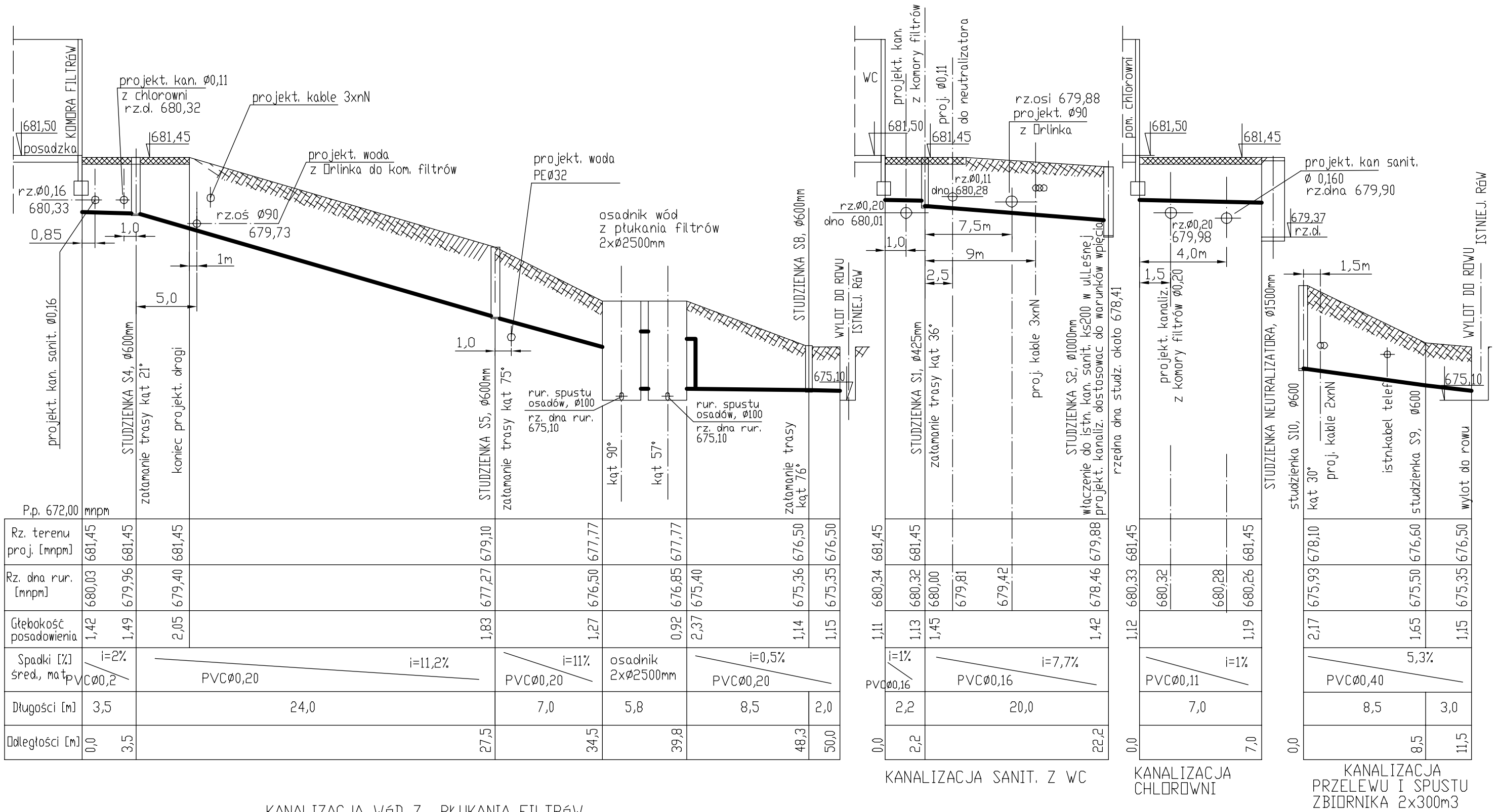
KANALIZACJA WÓD Z PŁUKANIA FILTRÓW
