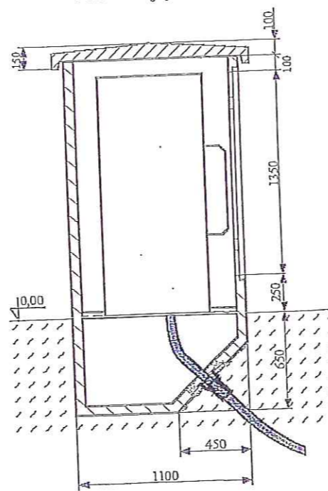
Przekrój pionowy
