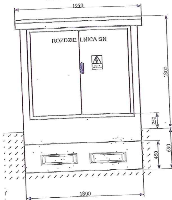
Elewacja frontowa
