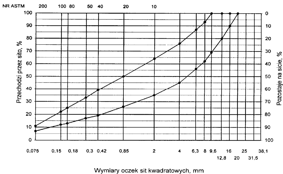
Rys. 2. Krzywe graniczne uziarnienia mieszanki mineralnej BA 0 do 12,8 mm do warstwy ścieralnej nawierzchni
