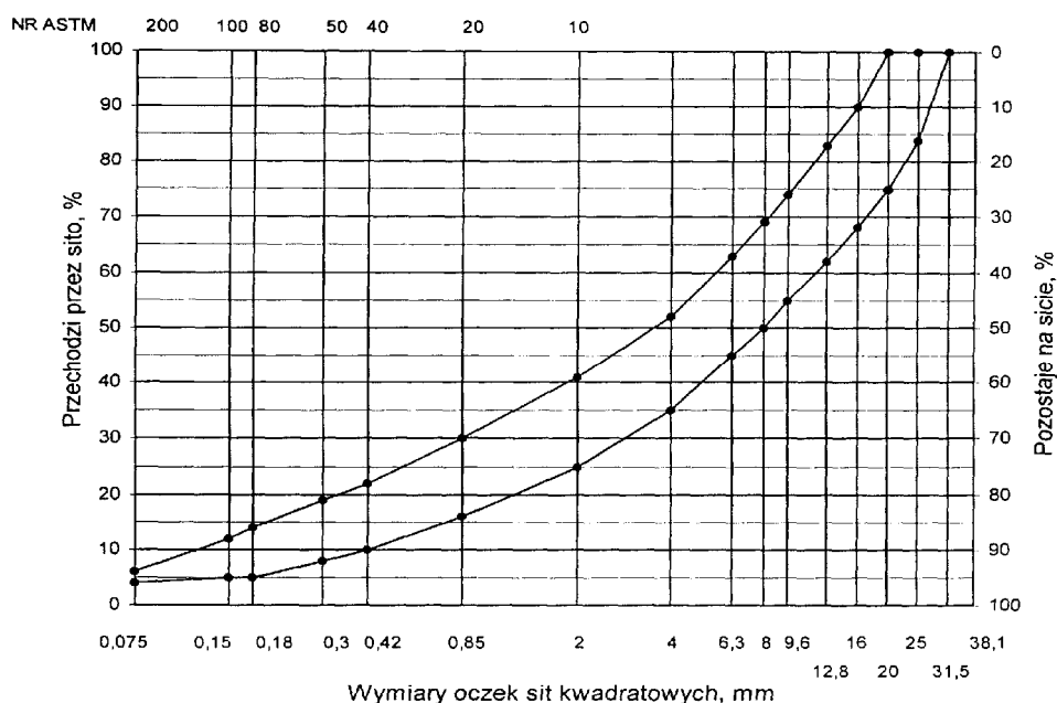
Rys. 2. Krzywe graniczne uziarnienia mieszanki mineralnej BA od 0 do 20 mm do warstwy wiążącej
