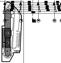
RZUT DACHU
