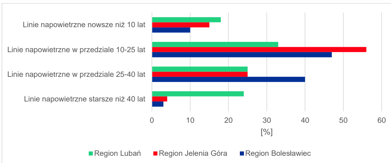
Ryc. 97 Charakterystyka wieku linii średnich napięć w rejonach obejmujących teren AJ
