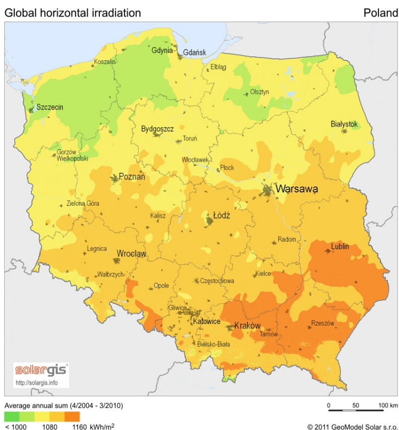
Rysunek 21. Natężenie promieniowania słonecznego w Polsce. (Źródło: http://solargis.info )
