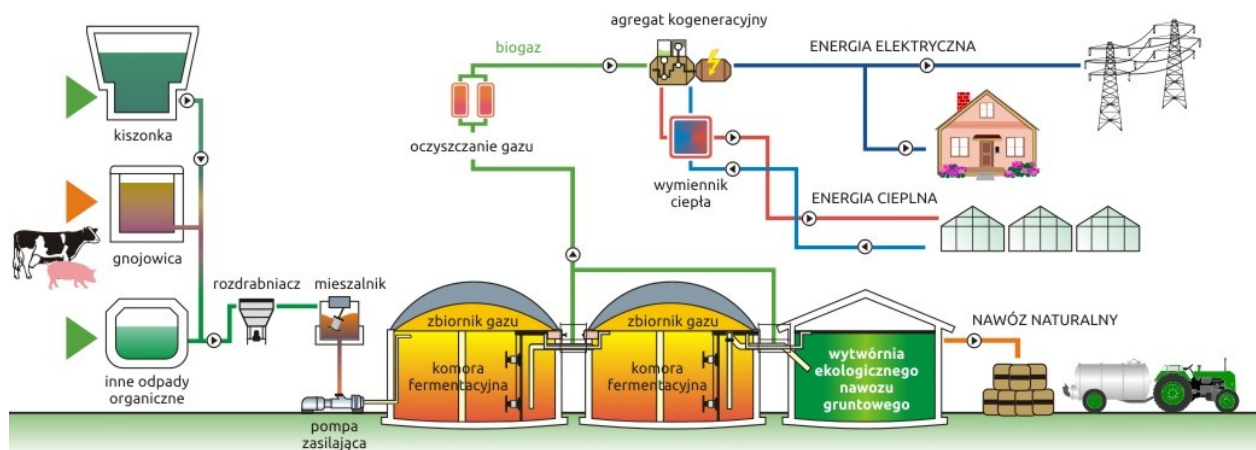
Rysunek 49. Schamat biogazowni
