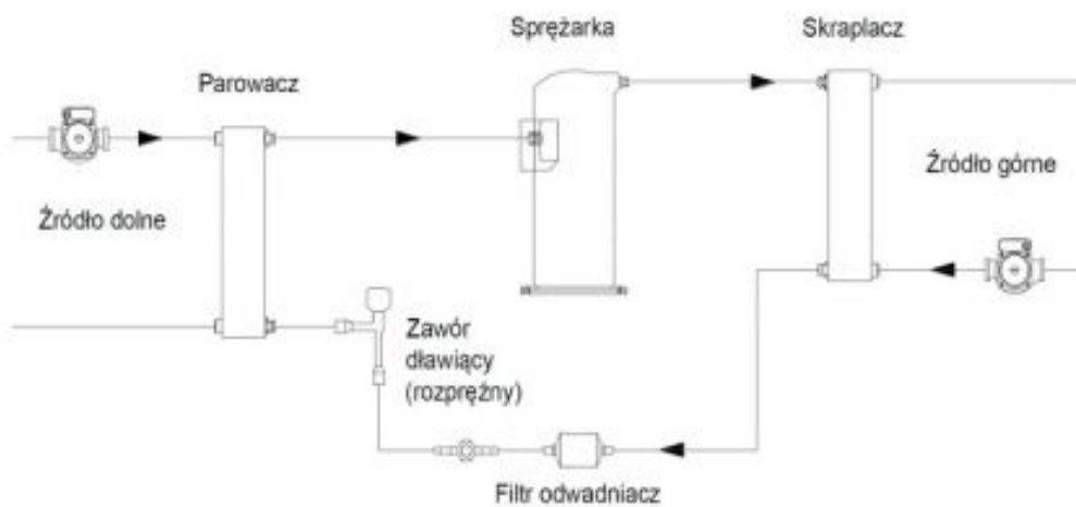
Rysunek 50. Pompy ciepła - zasada działania
