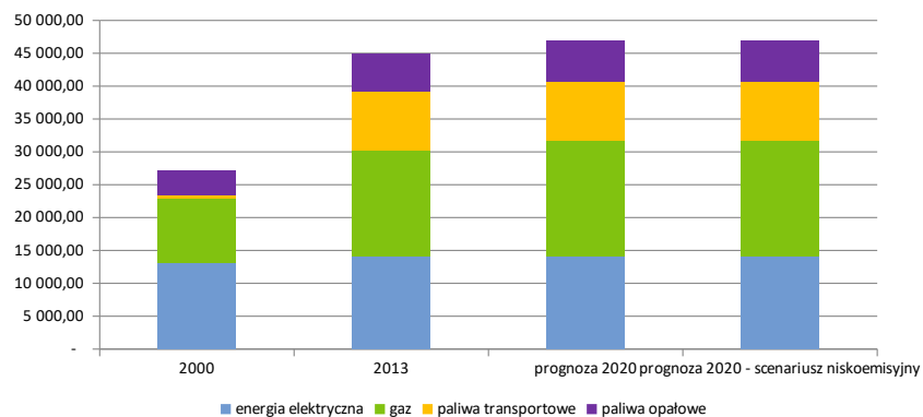
Bilans emisji [Mg CO 2 ]
