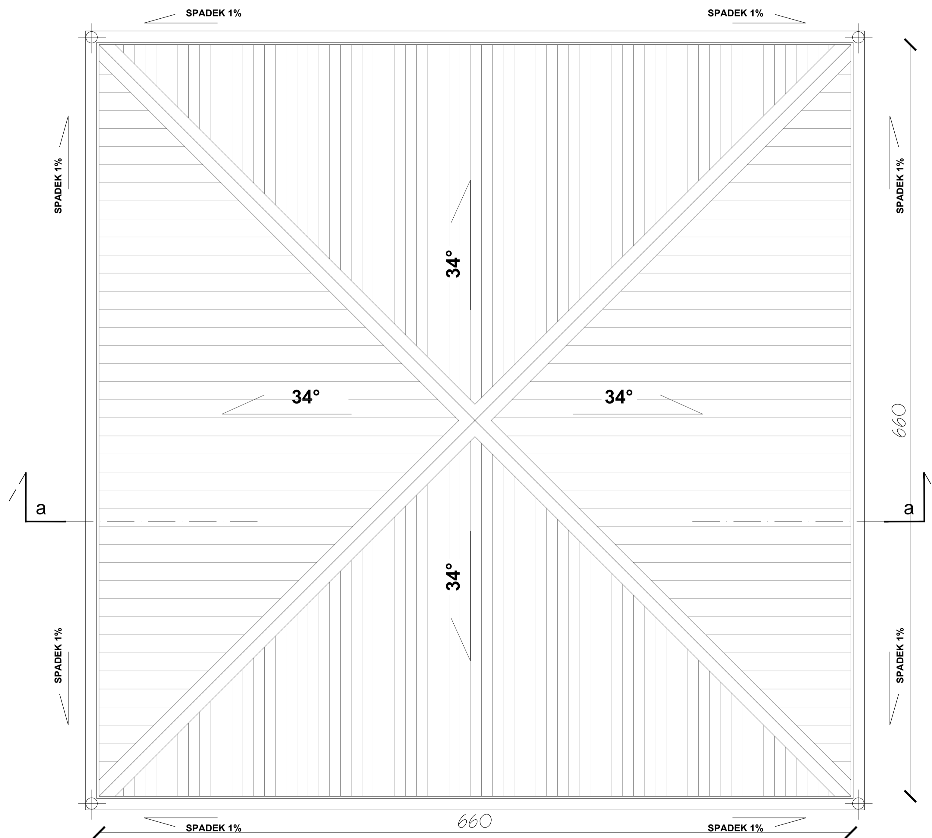
RZUT DACHU
