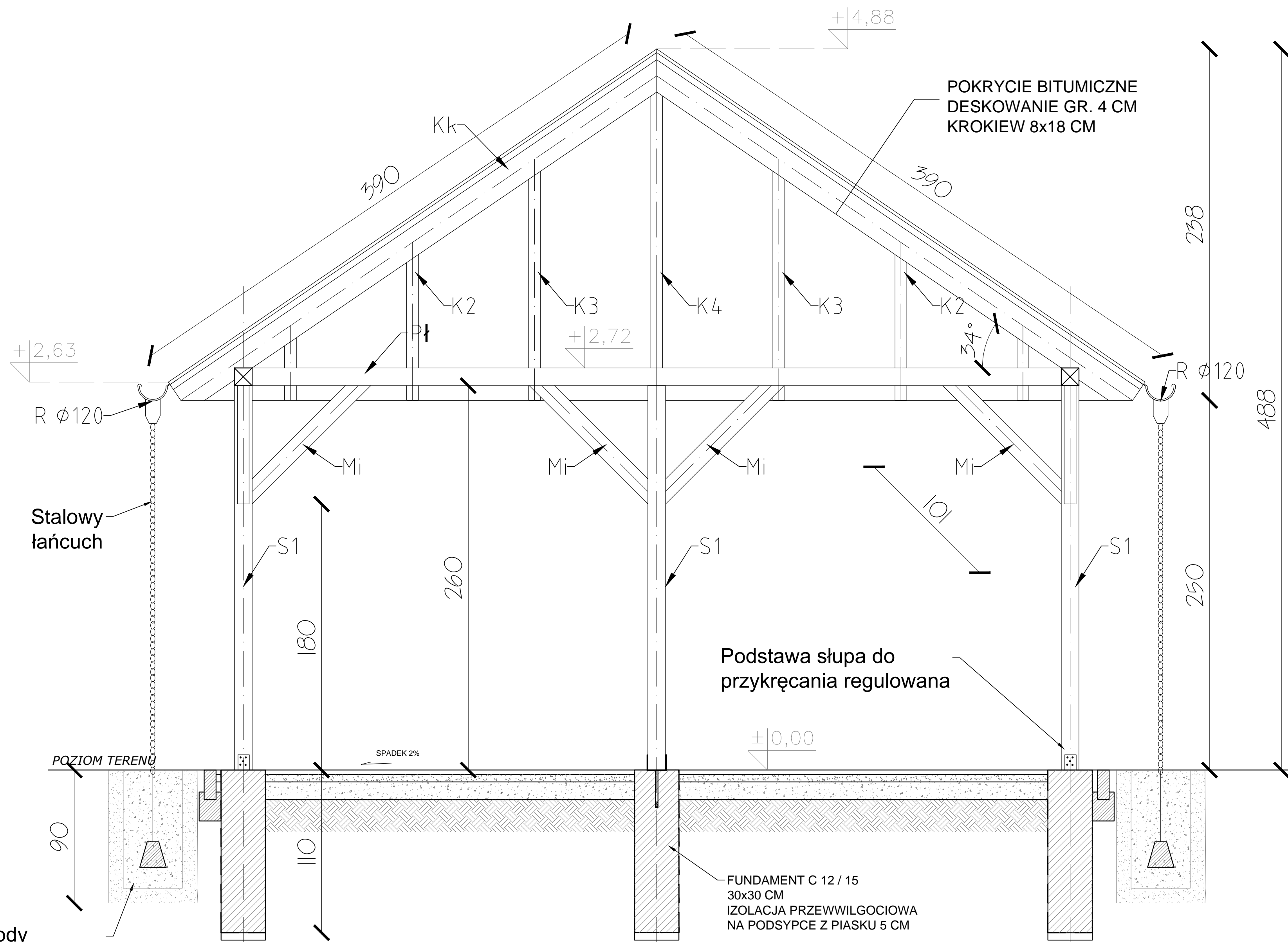
PRZEKRÓJ A - A
