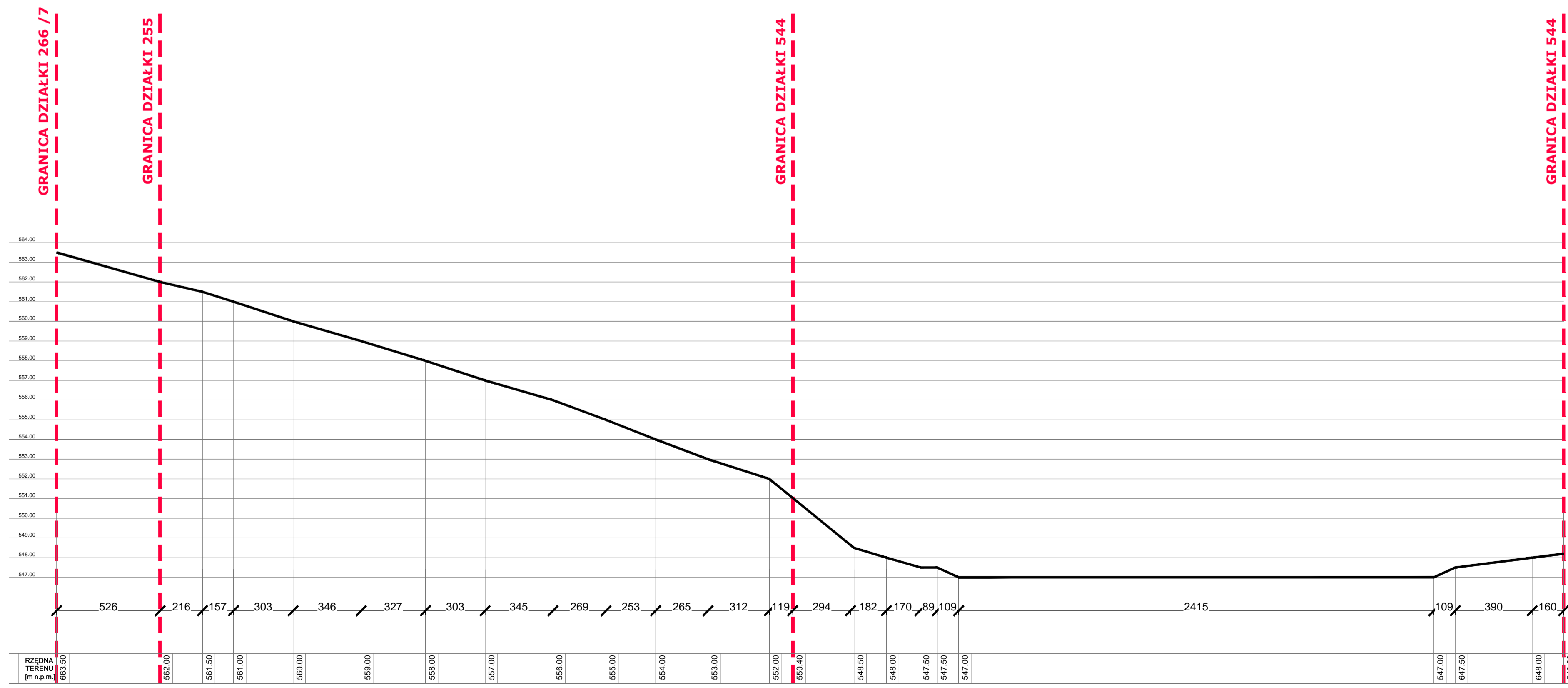
OGRÓD WODNY W KARPACZU STAN ISTNIEJĄCY - PRZEKRÓJ A-A SKALA 1:100
